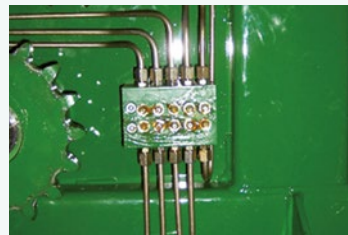
Zentral verrohrte Schmierleisten
